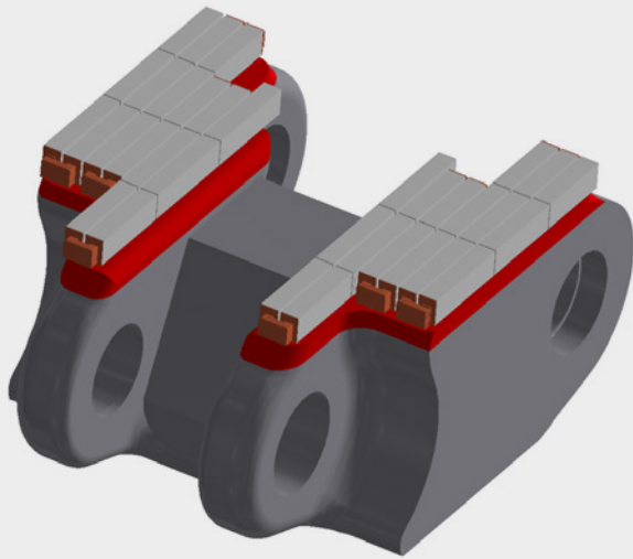
Bild 2: Kettengliedhärtung mit einem Gesamflächeninduktor – Härtezone rot dargestellt
