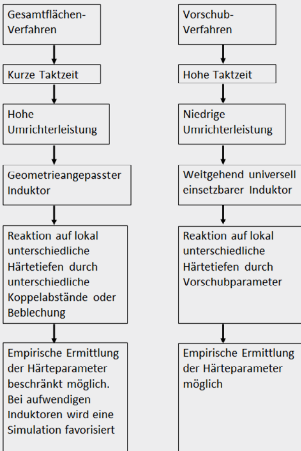
Bild 3: Gesamflächenverfahren vs. Vorschubverfahren
